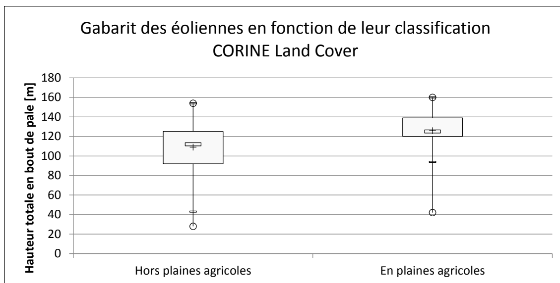
Figure 5 : Hauteur totale des éoliennes en fonction du type d'habitat
